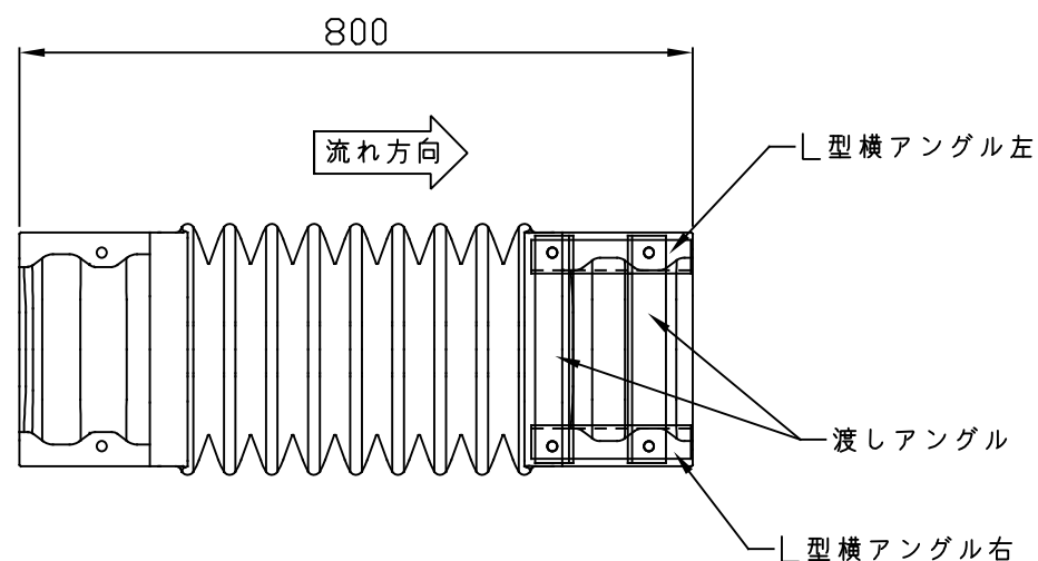
平面図
