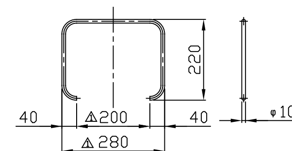
補強リング
