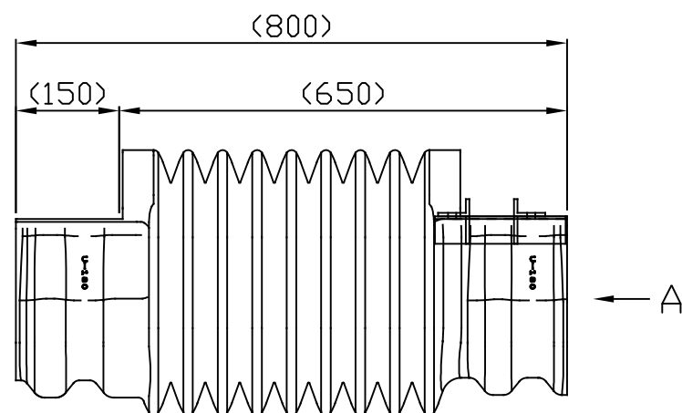
正面図
