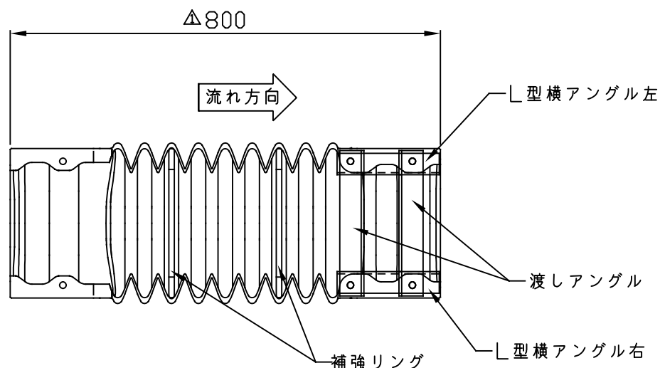
平面図
