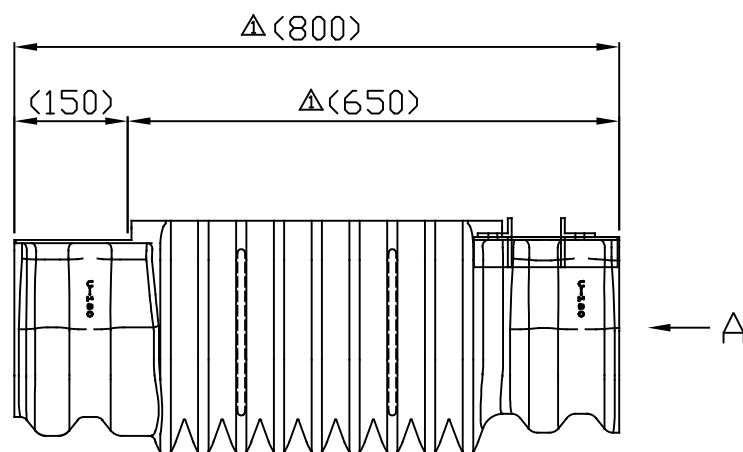
正面図
