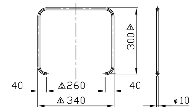
補強リング
