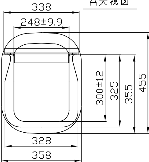
A矢視図
