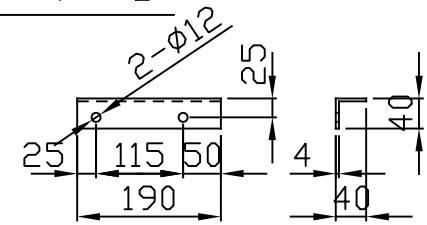
L型横アングル右
