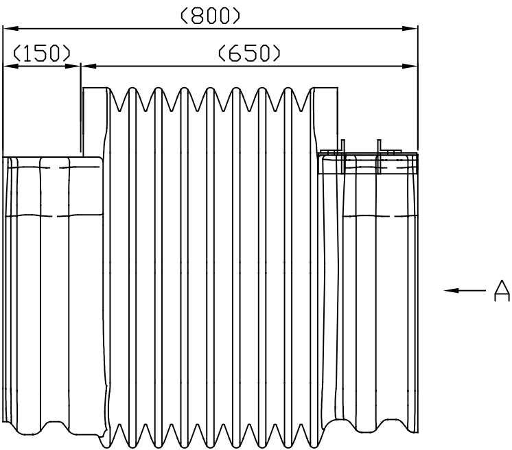
正面図
