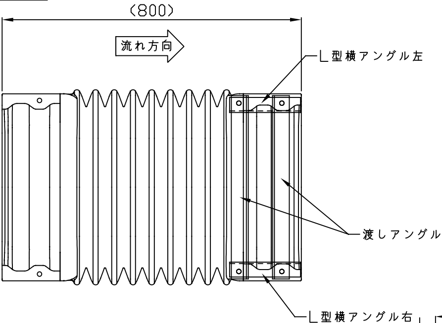
正面図
