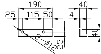
L型横アングル右
