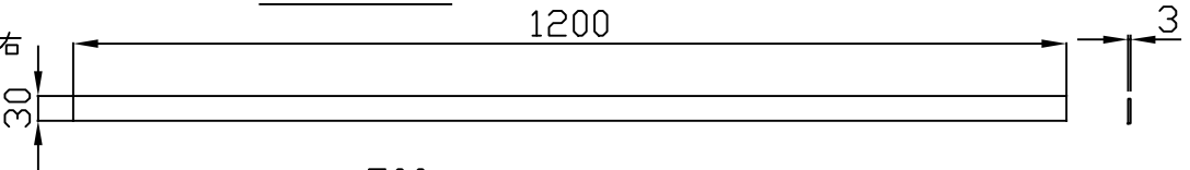
A矢視図
