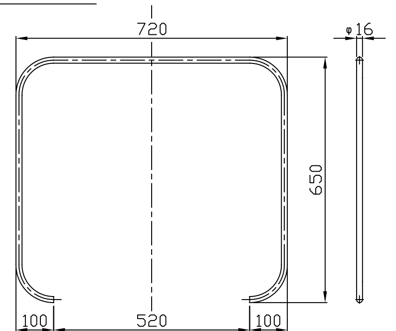
補強リング
