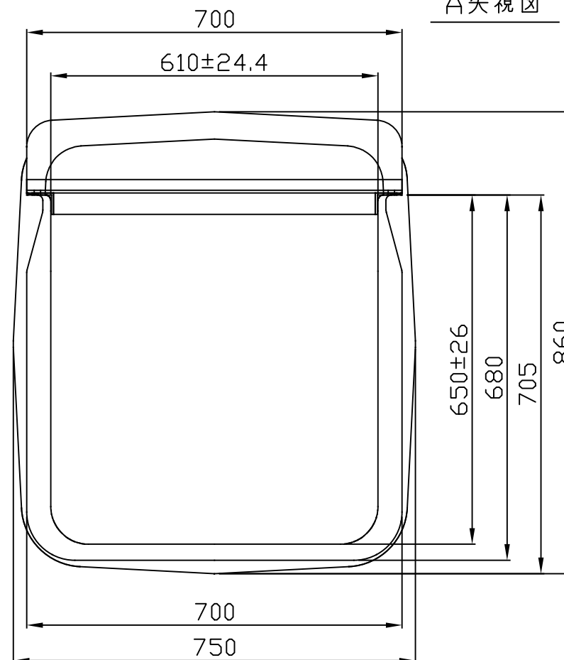
A矢視図
